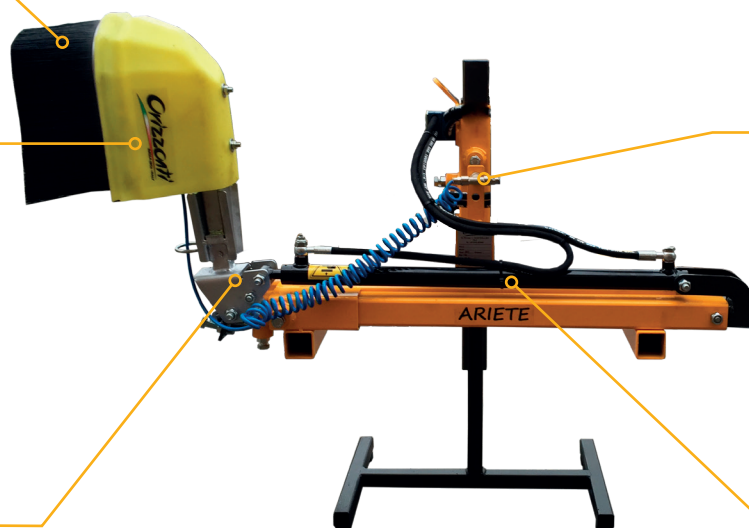
Martinetto per spostamento laterale con tubi ad innesti rapidi Hydraulic jack for lateral displacement with quick connections
